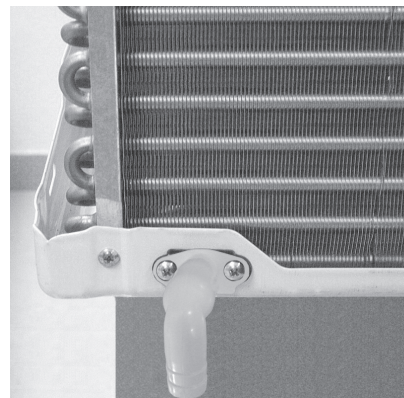
adaptador do dreno 2 Figura 3
